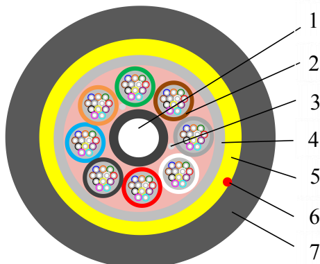
电缆截面示意图
