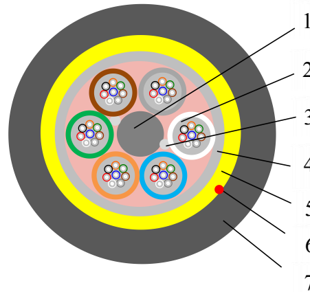
电缆截面示意图
