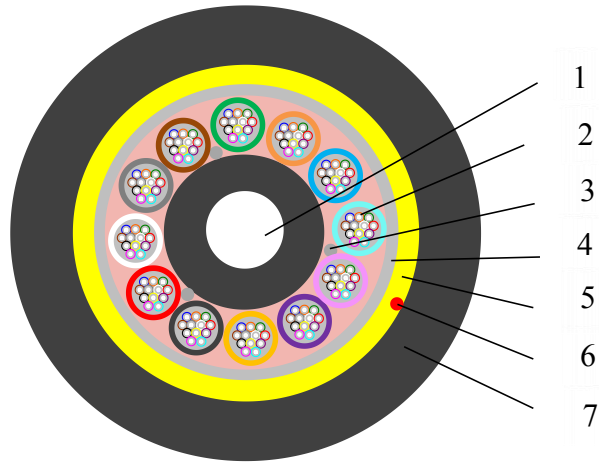
电缆截面示意图
